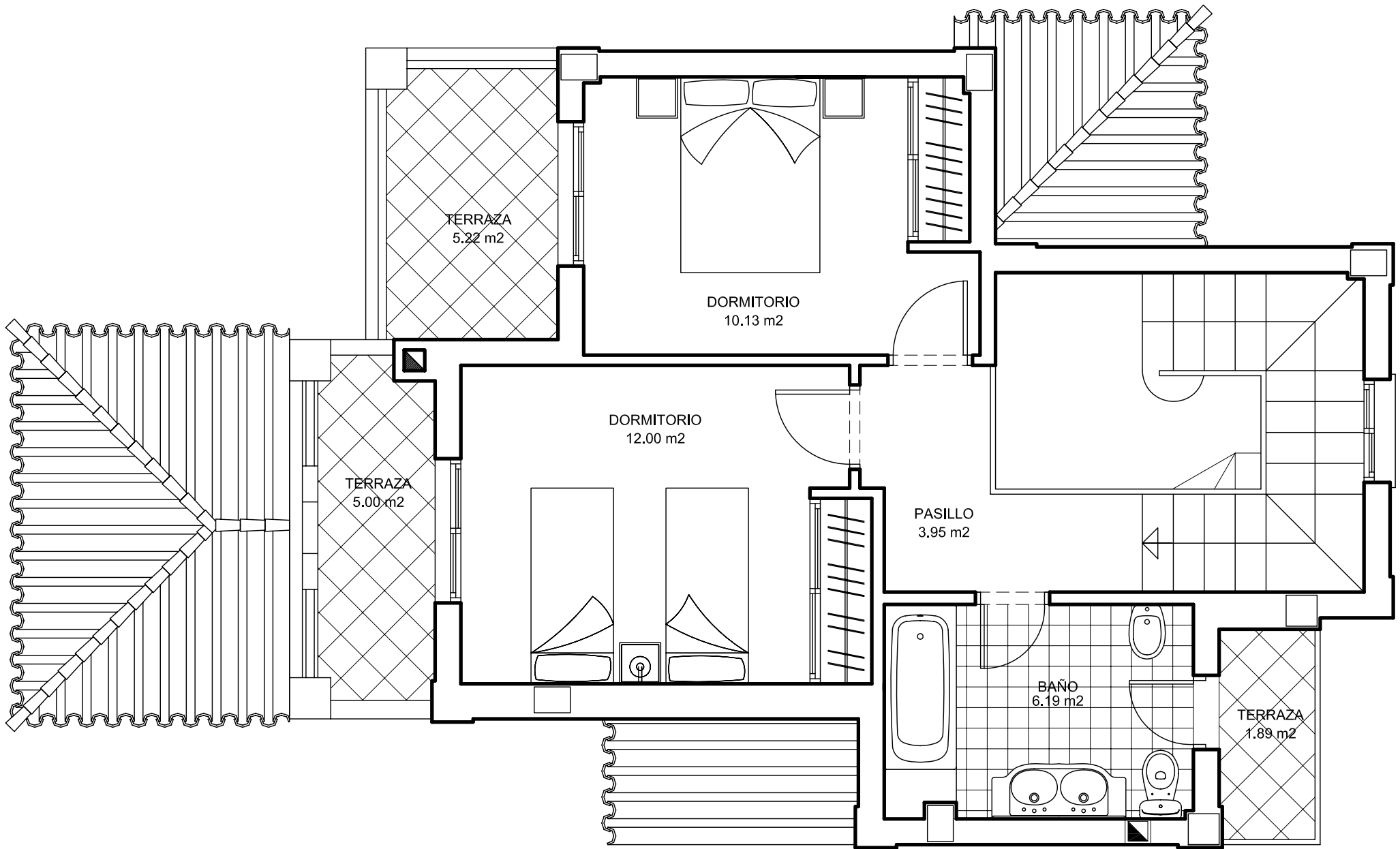
PLANTA PRIMERA
