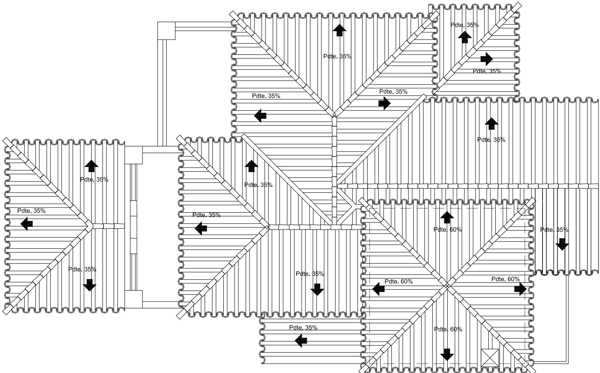
PLANTA CUBIERTA
