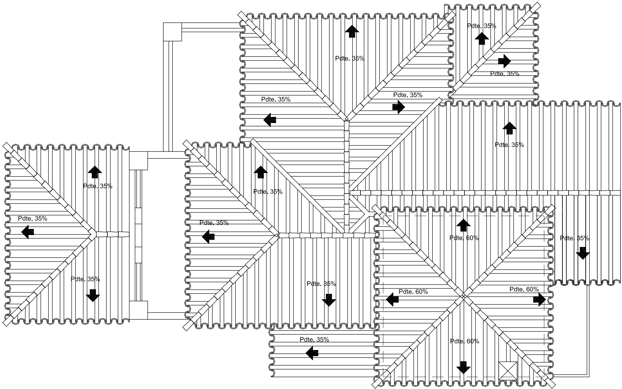
PLANTA CUBIERTA
