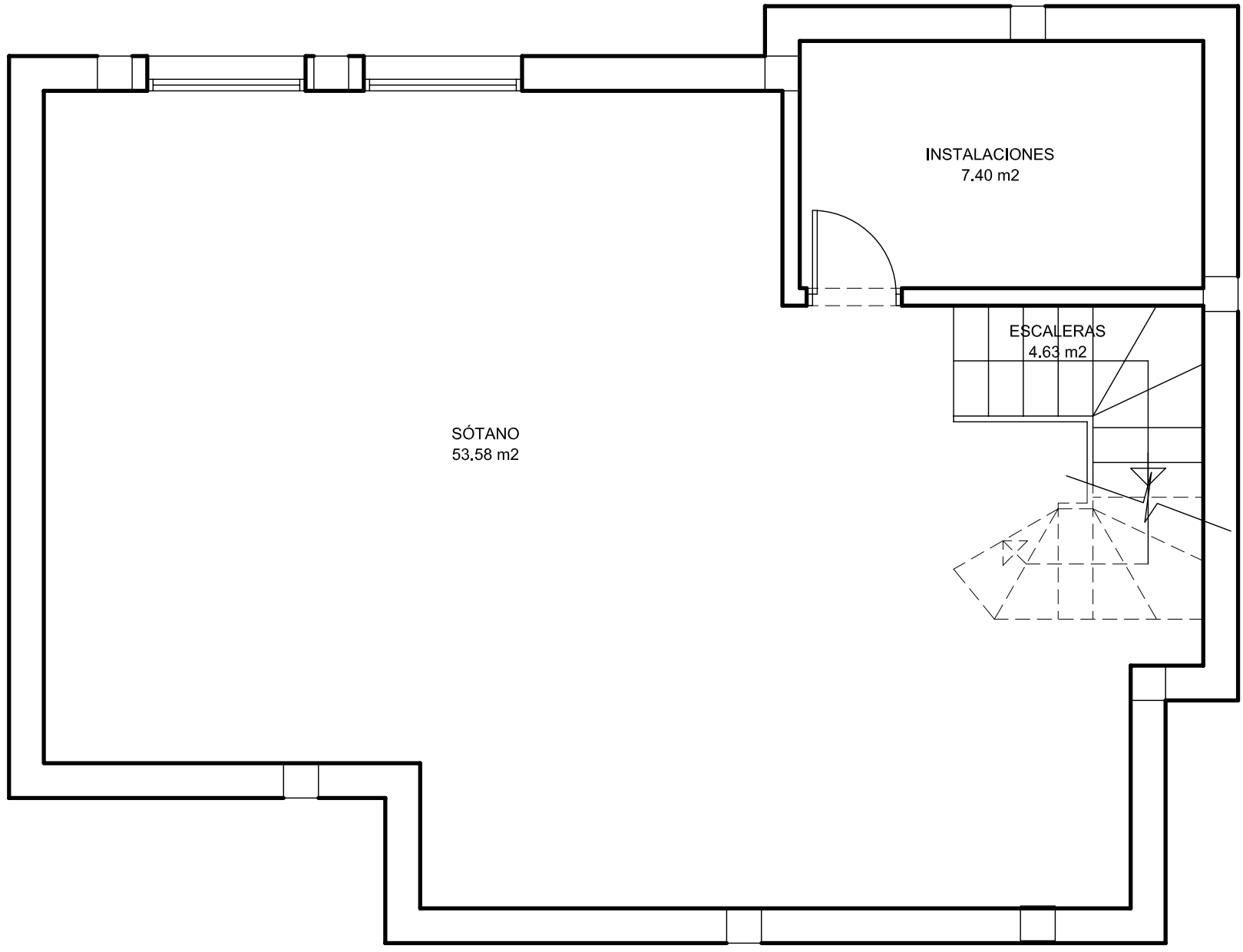
PLANTA SOTANO
