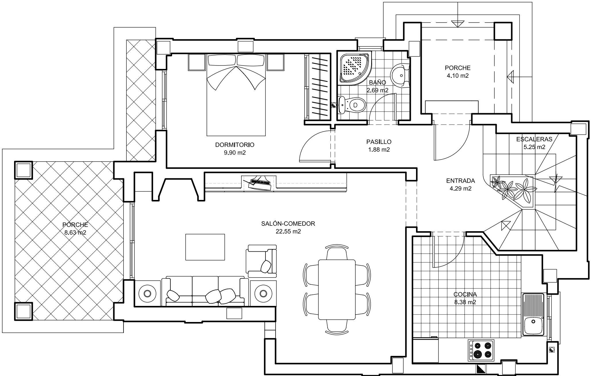
PLANTA BAJA
